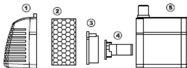
1) Filterabdeckung 2) Filter 3) Impellerabdeckung 4) Impeller 5) Pumpengehäuse
